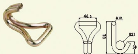
1-1/2' Double J Hook B/S: 6600lbs/3000kgs ArtNo. WH-038-01 N.W.: 0.18kg
